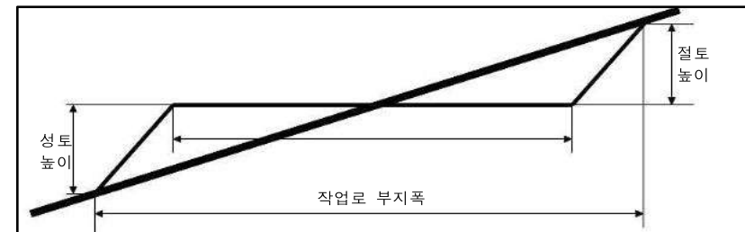
<작업로의 단면형태>
