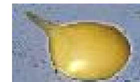
<뿌리혹선충(암컷)>
